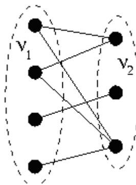
二分图
