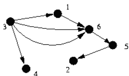
有向无环图
