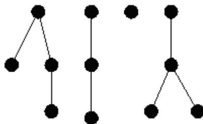
森林
