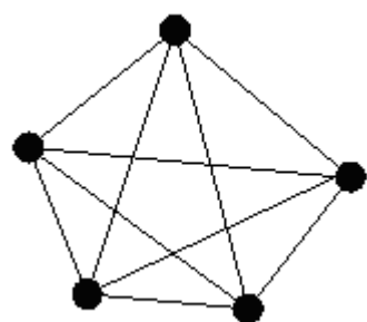
完全图
